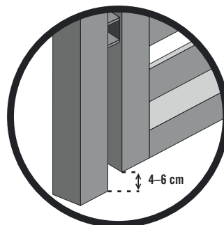
VZDIALENOSŤ KRÍDLA BRÁNY A BRÁNKY OD POVRCHU
