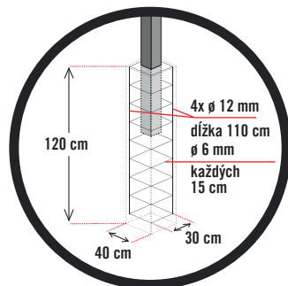
VYSTUŽENIE ZÁKLADOV STĽPIKOV
